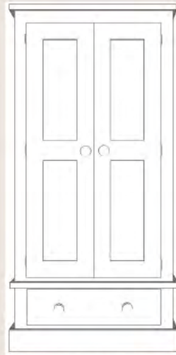
2 DOOR 1 DRW ROBE SU123 h:1860 w:900 d:595
