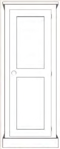
1 DOOR F/L ROBE SU120 h:1860 w:715 d:595
