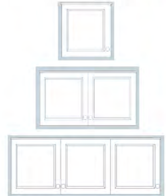
TOP BOXES h: 530 d: 545 1 DOOR SOM1DTOPBOX w: 480 2 DOOR SOM2DTOPBOX w: 915 3 DOOR SOM3DTOPBOX w: 1375
